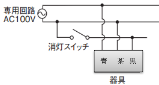
②常時消灯スイッチ付の場合
