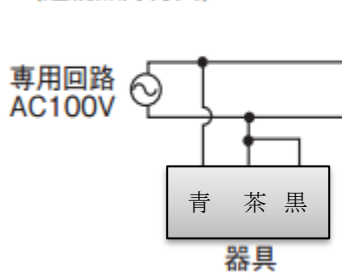
①常時消灯スイッチなしの場合 (連続点灯方式)
